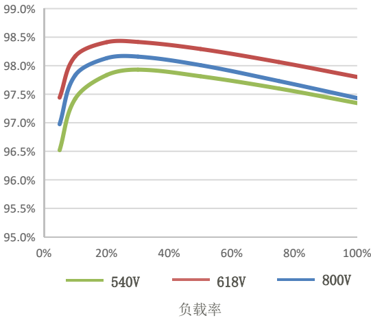
效率曲线
